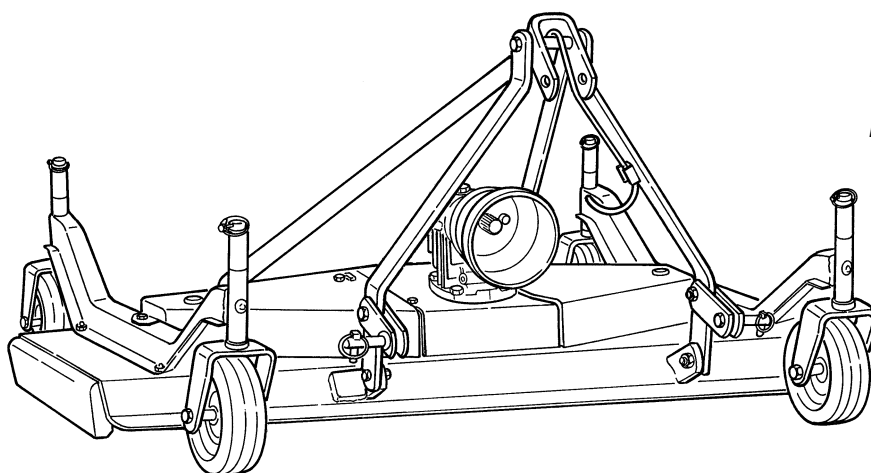
Fig. 4 Versione con attacco posteriore e con scarico laterale.
